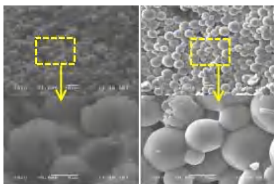
图 3 聚乳酸-氧化石墨基吡唑醚菌酯载药微球的酯微球在真菌菌丝和水稻根部的分布图
