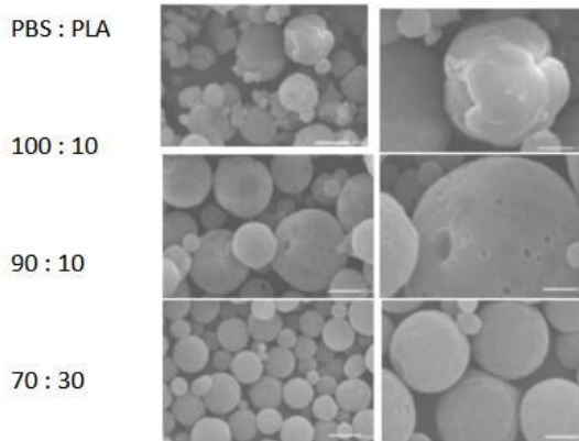
图 2 不同质量比醚菌酯·苯醚甲环唑 PBS/PLA 微球的 SEM 照片
