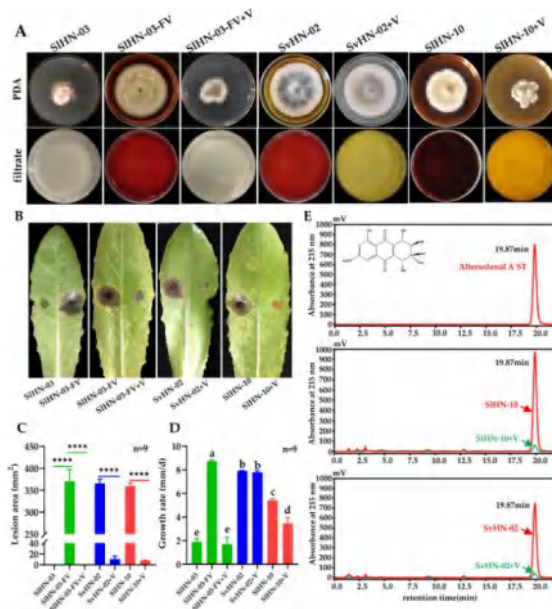
图 2 真菌病毒导致寄主弱毒力并降低寄主毒素 Altersolanol A 的合成
