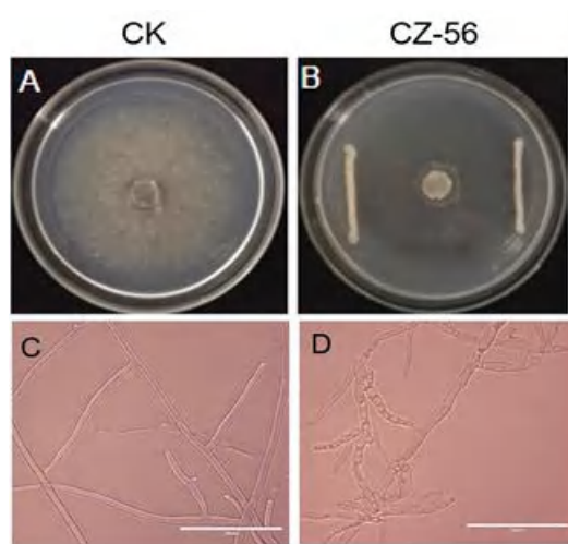
图 2 Pseudomonas mosselii CZ-56 平板抑菌效果及对靶斑病菌丝体的影响对比图
