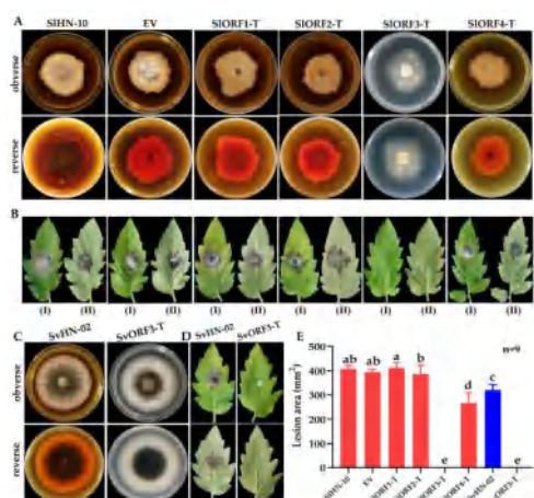
图3 病毒 ORF3 导致寄主弱毒力
