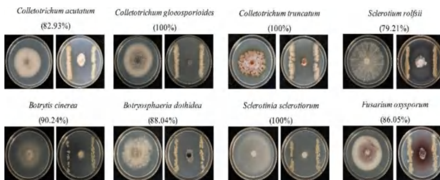
图 4 Streptomyces cinnamoneus ZZ-21 对果蔬上主要真菌病害的抑制效果
