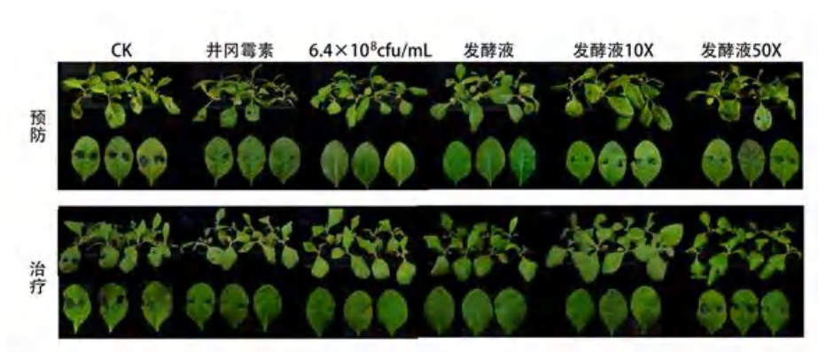
图 3 Pseudomonas mosselii CZ-56 不同处理对盆栽烟草接种烟草靶斑病菌的预防与治疗效果对比
