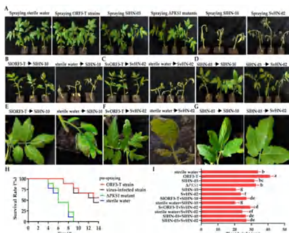
图4 喷洒转病毒 ORF3 的菌株的菌丝悬浮液可提高植物对强毒匍柄霉菌株的抗性
